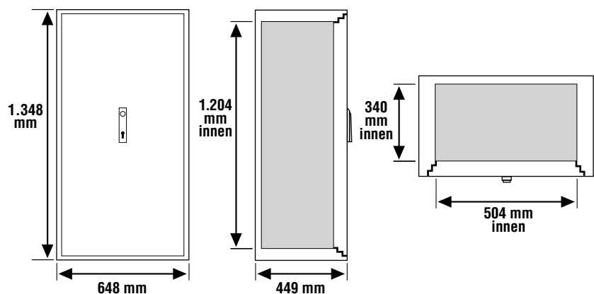
Frontalansicht
